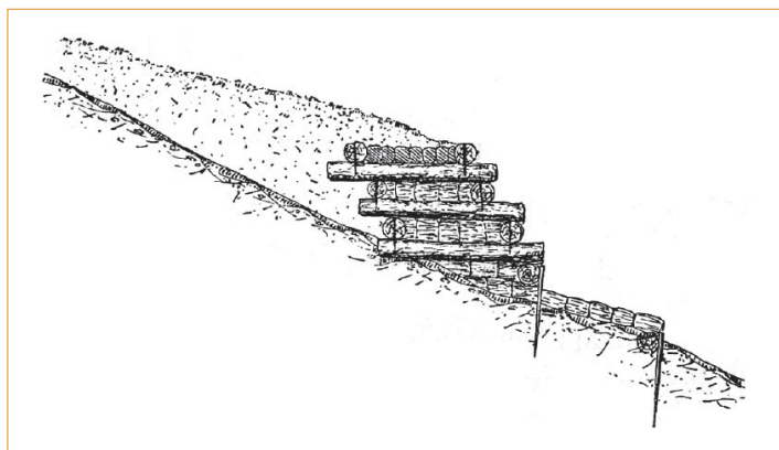
▲ Figure 5 – Barrages en bois avec fascines (Thiéry, 1891).
